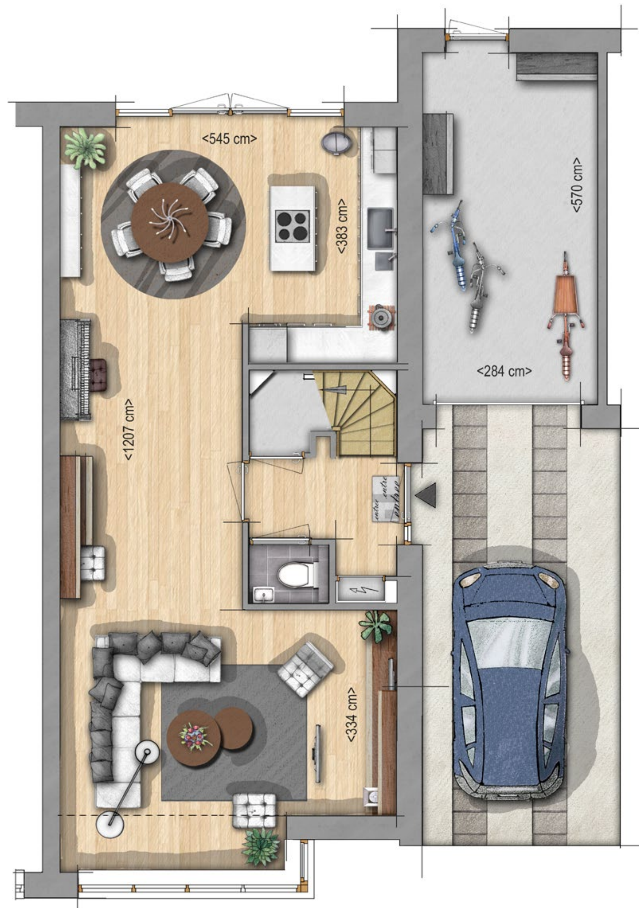
BEGANE GROND
